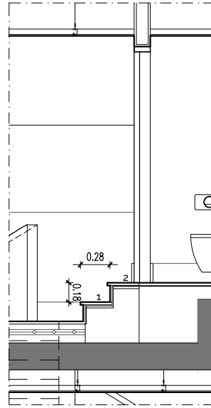
CORTE AA'
