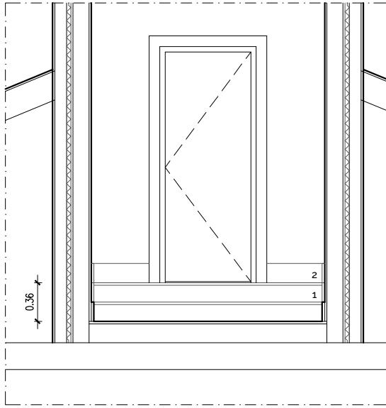
ALÇADO
