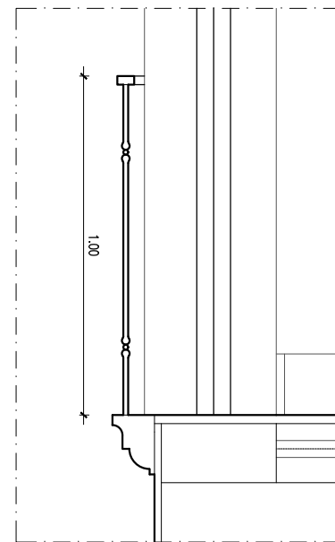
CORTE 1:20
