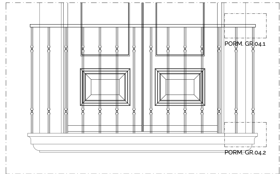
ALÇADO 1:20
