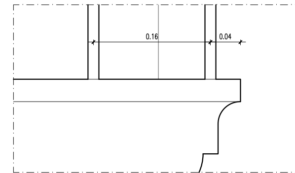
PORM. GR.04.2 1:5
