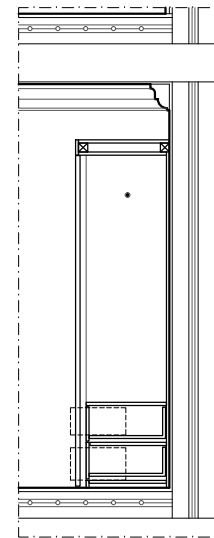
CORTE
