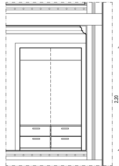
ALÇADO INTERIOR
