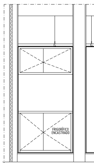
ALÇADO
