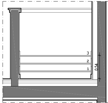
ALÇADO
